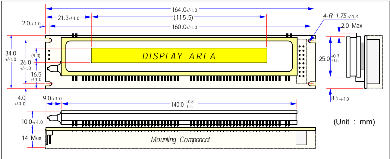
Fig-3. Outer Dimensions
